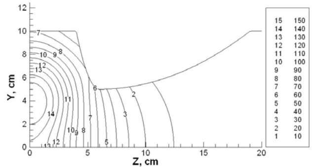
Рис. 10. Объемная плотность энергии излучения, 10^{-7} Дж/см 3 , \kappa = 1 \text{ см}^{-1}
